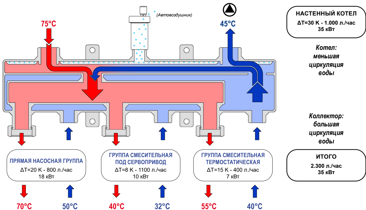
Пример функционирования коллектора с гидравлическим сепаратором
