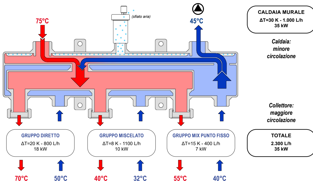
Esempio di applicazione del collettore compensatore
