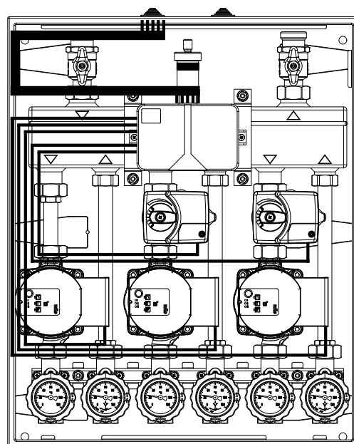
Percorso raccomandato per i cablaggi
