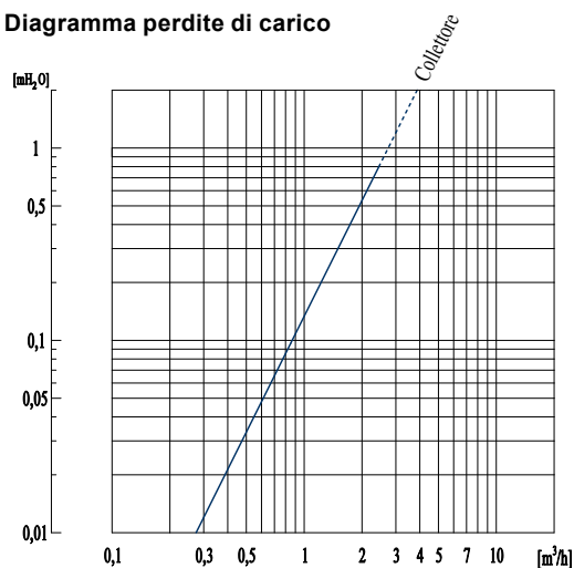
Diagramma perdite di carico
