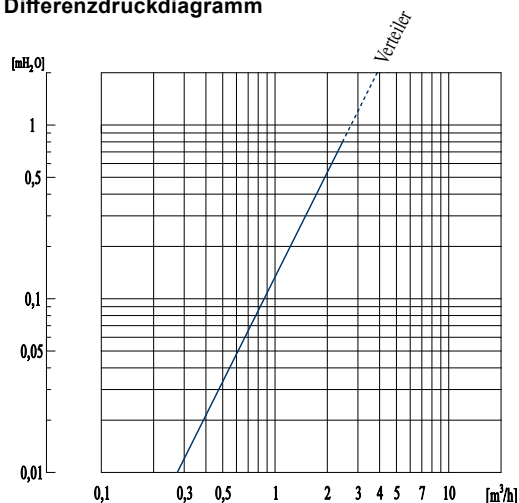
Differenzdruckdiagramm
