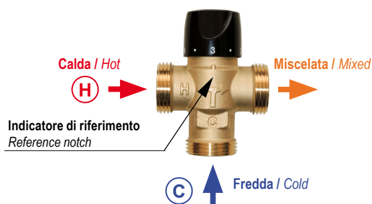
Art. 729 Con valvole di non ritorno. With check valves.
