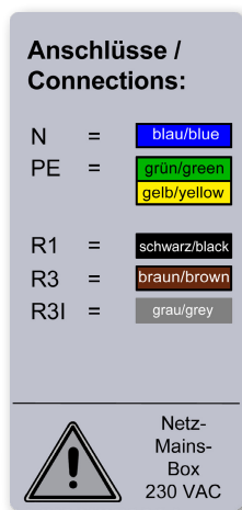
Illustration 3: Connexions à la boîte à relais
