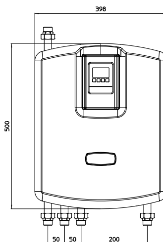
III.3: Encombrements et entraxes significatifs du module
