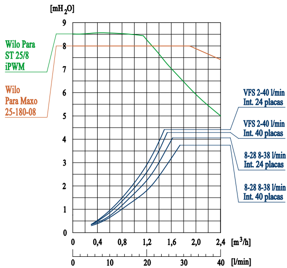
Curvas características del circuito solar.
