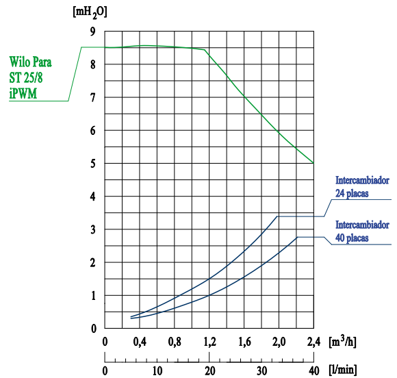
Curvas características del circuito secundario.
