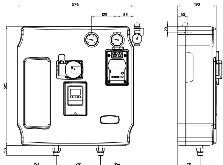
Abb. 3: wichtige Maße und Achsabstand der Station
