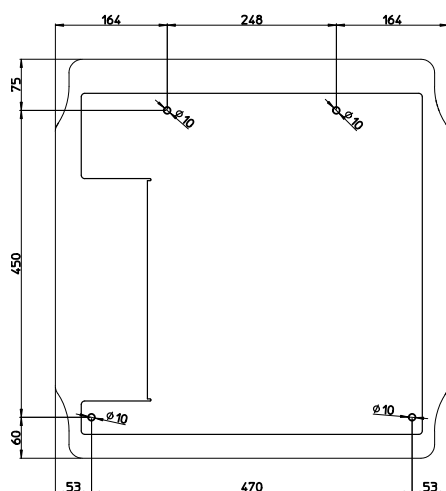
Illustration 2 : plaque derrière la coque isolante pour l'installation au mur du module.
