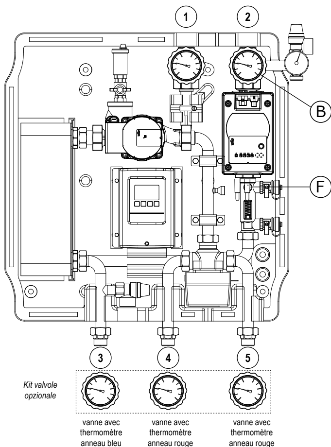
Illustration 1 : Schéma des connexions et du kit vannes optionnel
