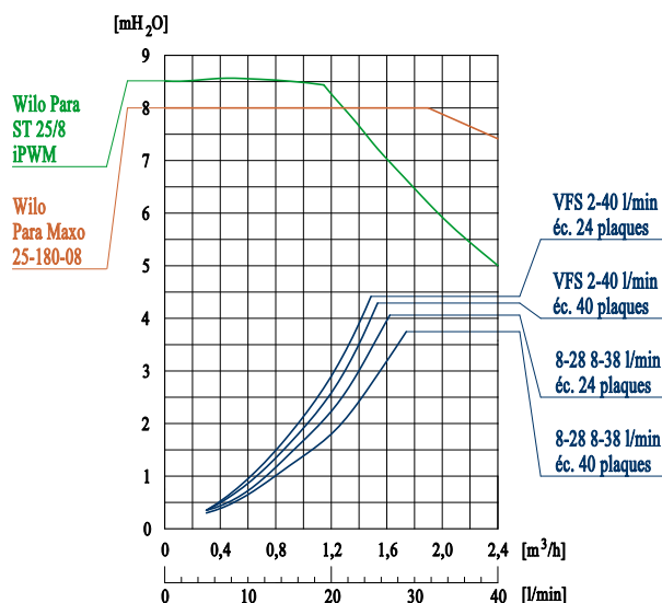
Courbes caractéristiques du circuit solaire
