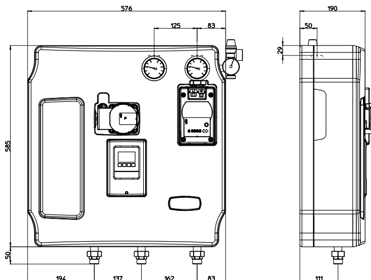
Illustration 3 : dimensions et entraxes significatifs du module.
