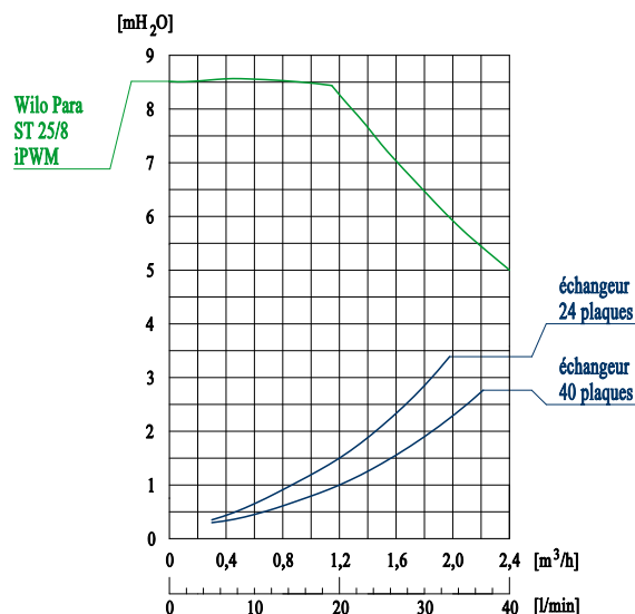
Courbes caractéristiques du circuit secondaire
