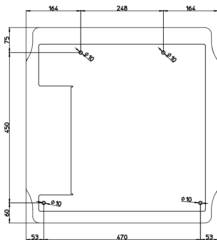
Abb. 2: rückseitige Metallplatte für die Wandmontage der Station
