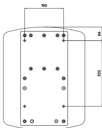
Illustration 2: plaque métallique dans le derrière de la coque isolante pour la fixation au mur du module.
