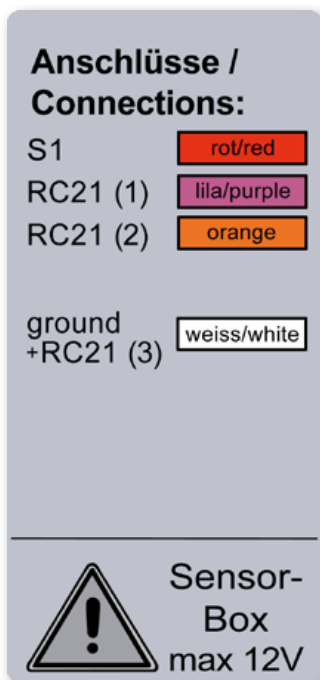
Abbildung 1: Anschluss der Fühler an die „Sensor Box“
