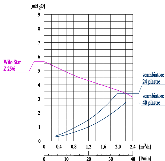
Curve caratteristiche circuito secondario (ACS)
