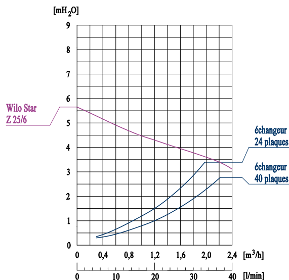
Courbes caractéristiques du circuit secondaire (ECS)
