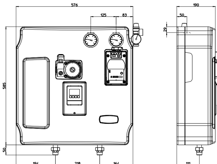
Illustration 3 : dimensions et entraxes significatifs du module.
