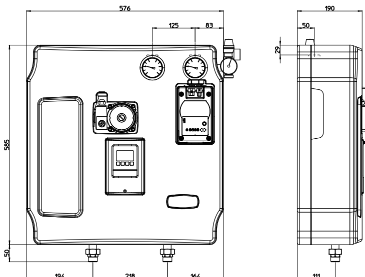
Figura 3: dimensiones totales y distancias significativas del módulo.
