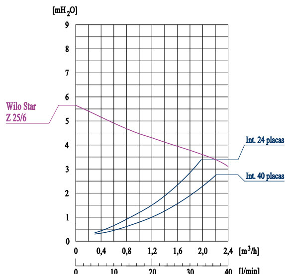
Curvas características del circuito secundario.
